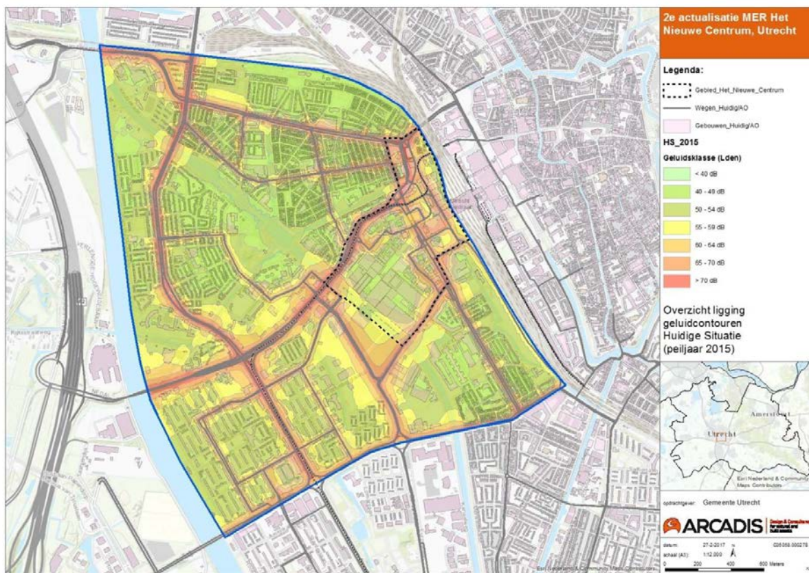
Figuur 9 Berekende geluidscontouren Huidige Situatie, peiljaar 2015
